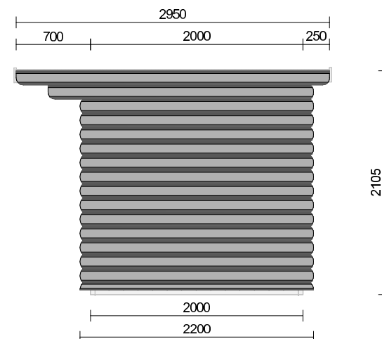
parete04
